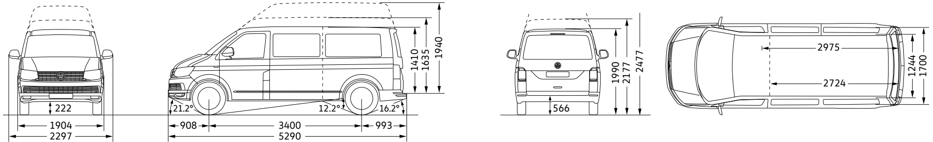
LWB Van*
